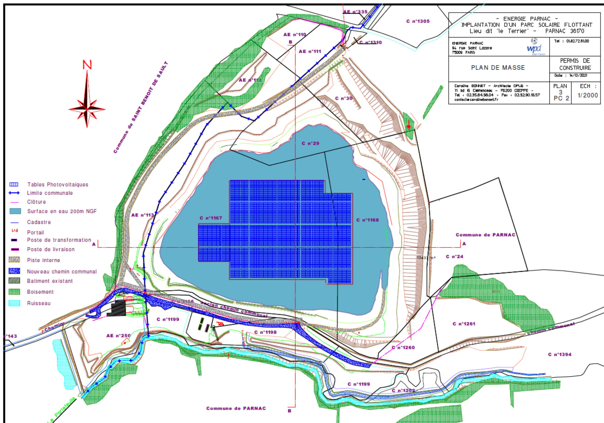
Figure 9 : Plan de masse (Source : WPD)
